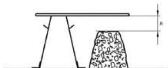
Рисунок 1 — Измерение осадки
