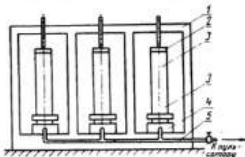
Схема испытательной машины на три образца
