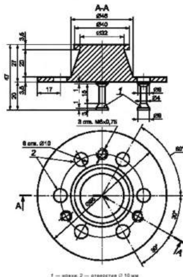
Рисунок 3 — Прибор Красного
