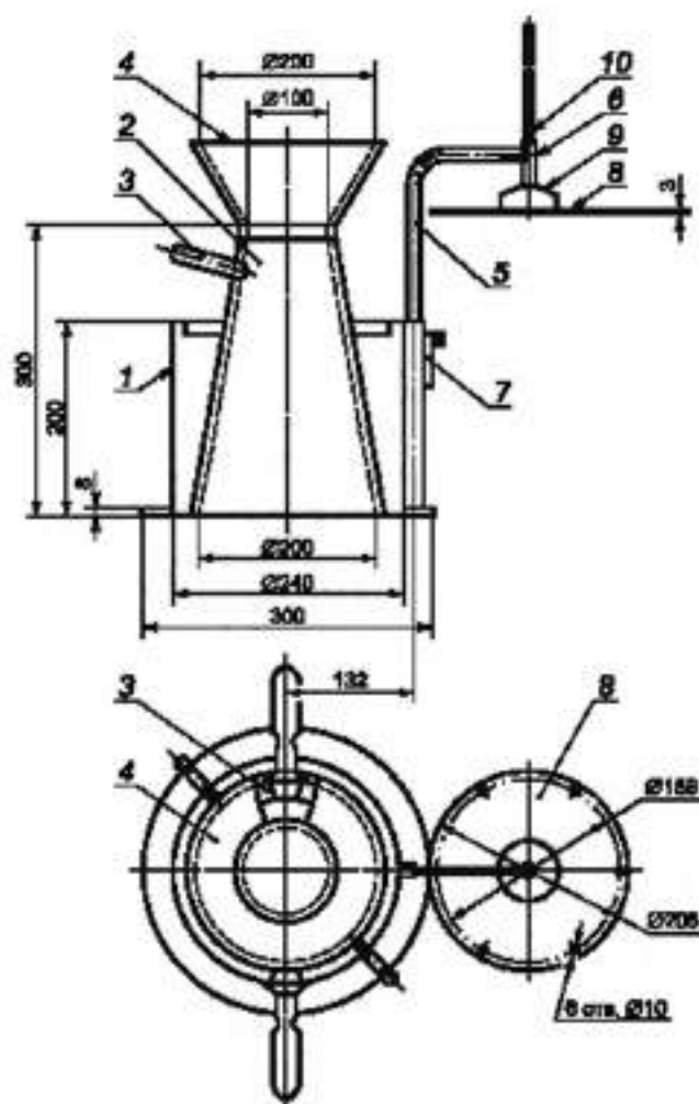
1 — цилиндр с фланцем в основании; 2 — конус; 3 — кольцо-держатель с ручками; 4 — загрузочная воронка; 5 — штырь; 6 — направляющая втулка; 7 — фиксирующая втулка; 8 — диск с шестью отверстиями; 9 — стальная шайба; 10 — штырь
