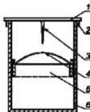
1 — крышка; 2 — ограничители; 3 — стрелка; 4 — лотки; 5 — прижимающий плавник; 6 — цилиндрический сосуд
