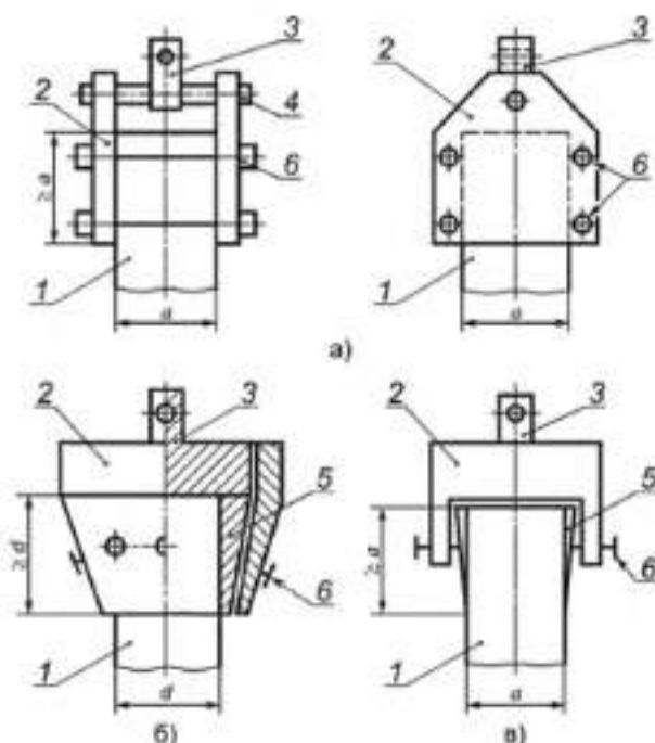
1 — образец, 2 — захват, 3 — концевой элемент шарнира Гуха, 4 — ось, 5 — цапга, 6 — стягивающие винты
