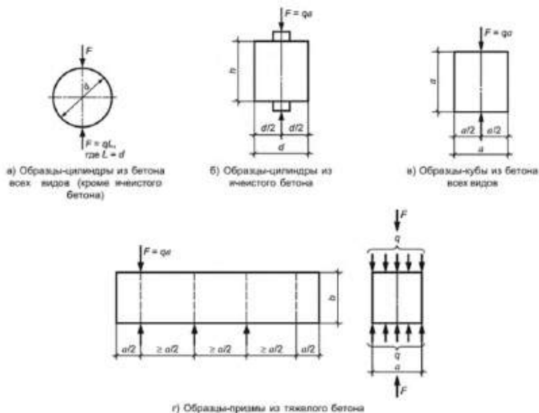
Рисунок 3 — Схемы испытания на растяжение при раскалывании
