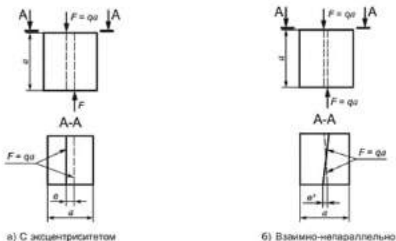
Рисунок 4 — Погрешности расположения плоскостей действия нагрузок при испытании на растяжение при раскалывании
