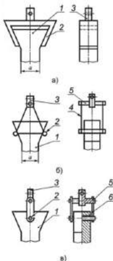
1 — образец, 2 — захват, 3 — концевой элемент шарнира Гукса; 4 — гибкая тяга, 5 — ось; 6 — жесткая тяга
