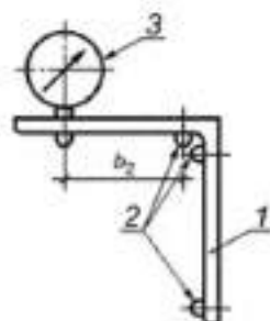
b_2 — база прибора; 1 — корпус (угольник); 2 — опоры; 3 — индикатор
