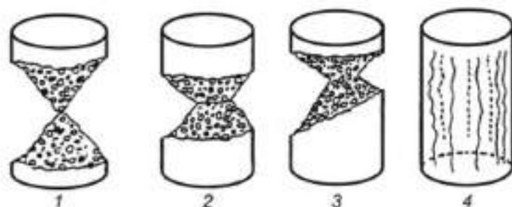
Рисунок Е.3 — Удовлетворительные разрушения образцов-цилиндров
